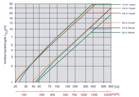
Diagram 15, kastelengde Tellus-LØV-S, isotherm
